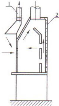
图 12 补风罩
