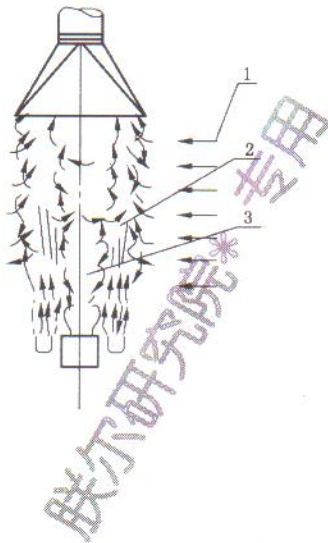
图 11 气幕隔离罩
