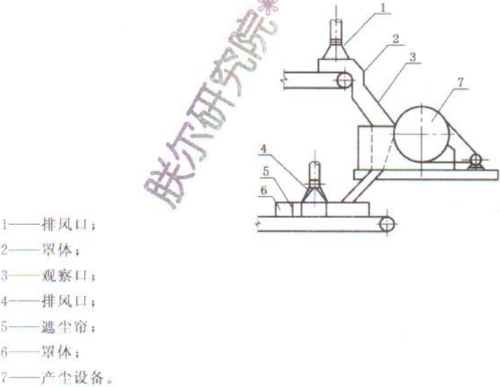
图 1 局部密闭罩
