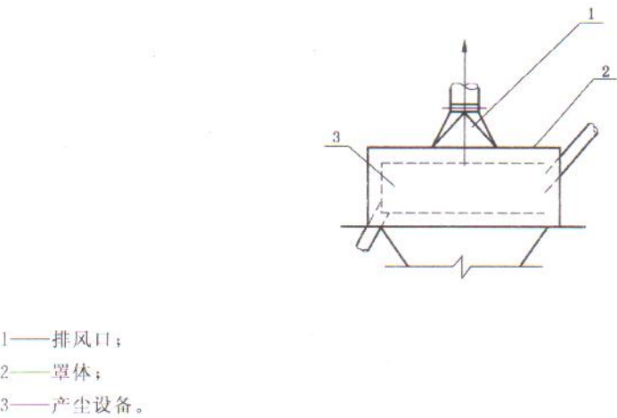
图 2 整体密闭罩
