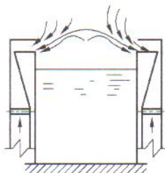
图 8 槽边罩
